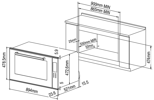
PPOV-9S-48
